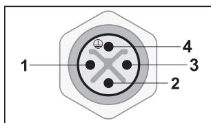
Schemazeichnung M12 S-kodiert
